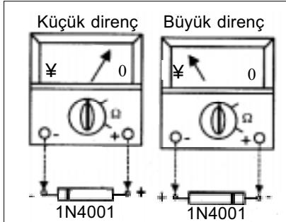
Şekil 3.15: Diyotların sağlamlık testinin analog ohmmetreyle yapılışı
