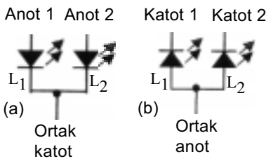
Şekil 3.33: Çok renkli led diyotların yapısı ve çok renkli led örnekleri
