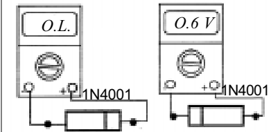
Şekil 3.16: Diyotların sağlamlık testinin polarma gerilimine bakarak yapılışı
