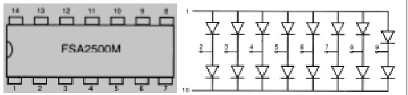
Şekil 3.62: Entegre tipi diyotlar
