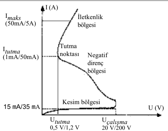
Şekil 3.59: Dört tabaka diyotların elektriksel karakteristik eğrisi
