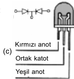
Şekil 3.33: Çok renkli led diyotların yapısı ve çok renkli led örnekleri
