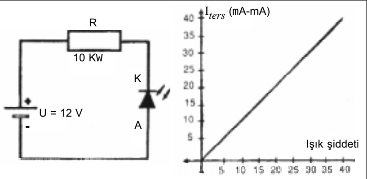
Şekil 3.65: Işığa bağlı olarak foto diyotların üzerinden geçen akımın eğrisi
