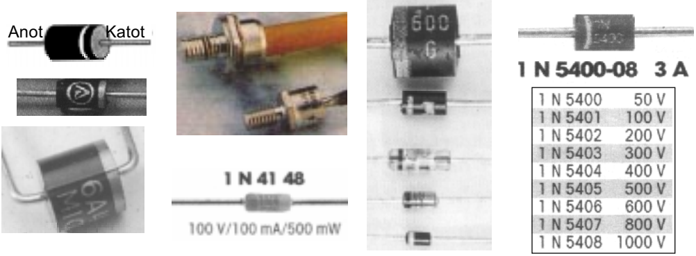
Şekil 3.14: Uygulamada kullanılan çeşitli doğrultmaç diyotları
