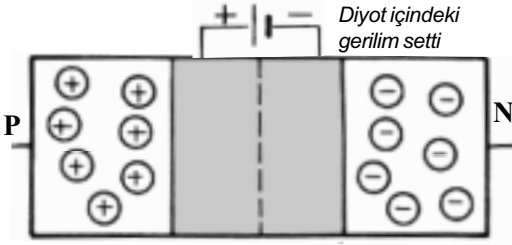
Şekil 3.9: Diyotların ilettime geçme geriliminin ana üretece ( U_{CC} ) ters bağlı pil gibi gösterilişi
