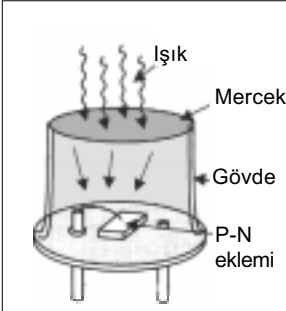
Şekil 3.64: Foto diyotların yapısı
