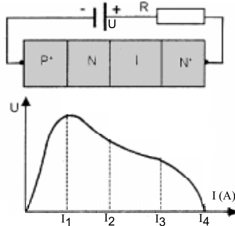
Şekil 3.48: İmpatt diyotların yapısı ve elektriksel karakteristik eğrisi
