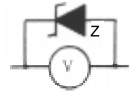
Şekil 3.29: Ölçü aletlerinin zener diyot ile yüksek gerilimden korunması
