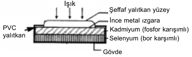
Şekil 3.71: Foto pillerin yapısı
