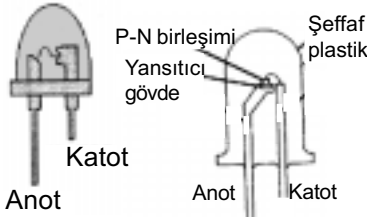
Şekil 3.31: Çeşitli led diyotlar
