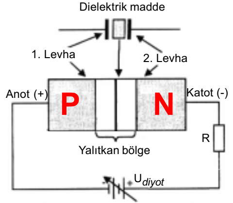
Şekil 3.36: Kapasitif diyotların ters polarize edilmesi
